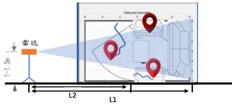
图 6 水平安装示意图
