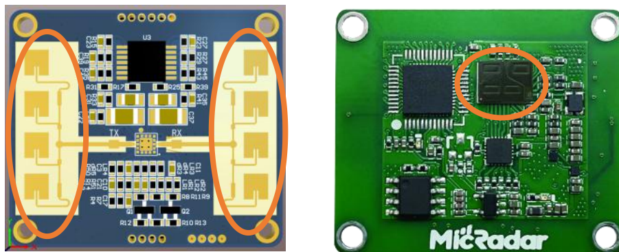
黄色住部分为雷达天线
